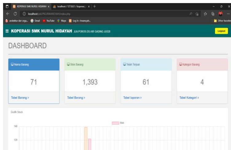
Gambar 3.9 Desain Halaman
