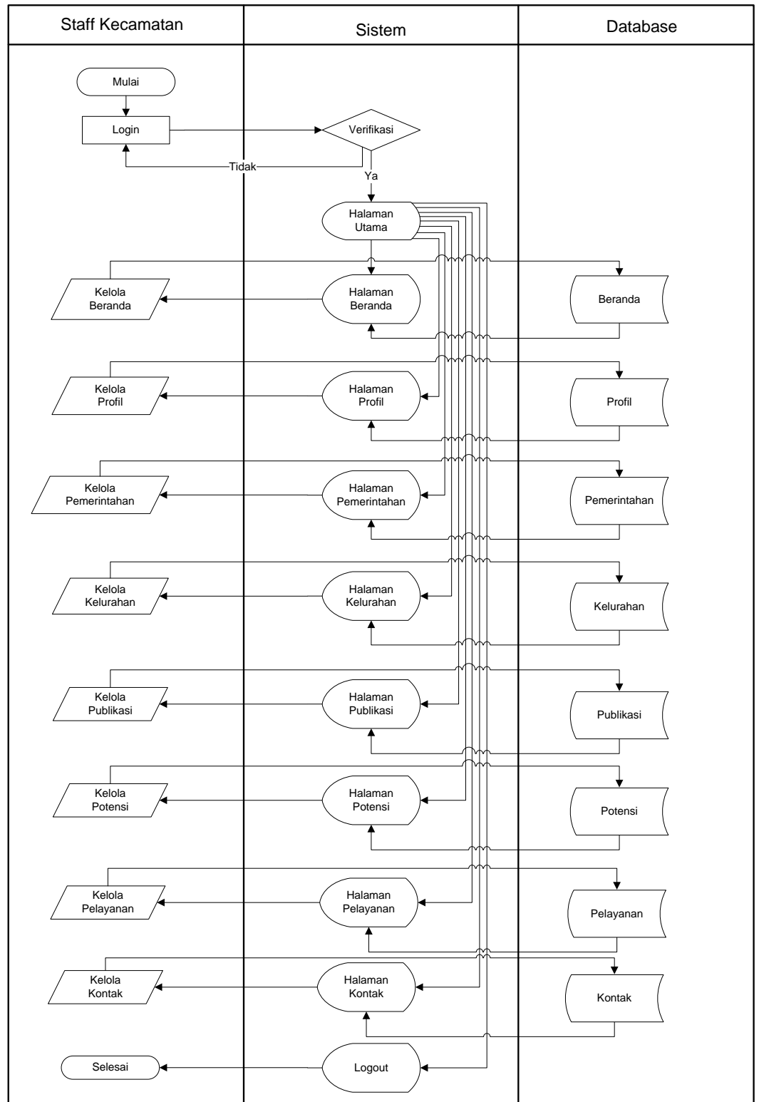
Gambar 5.14. Flowchart yang diusulkan
