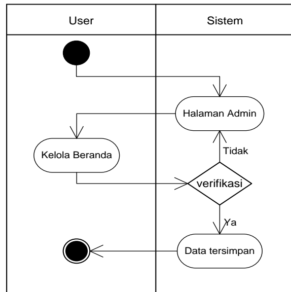
Gambar 5.5. Activity Diagram Kelola Beranda
