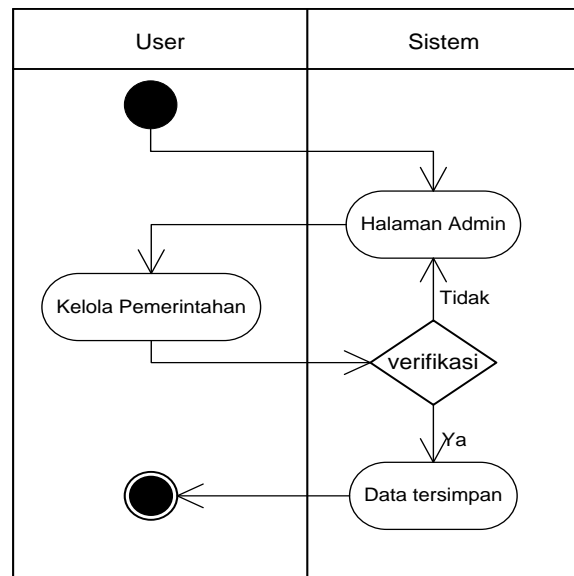
Gambar 5.7. Activity Diagram Kelola Pemerintahan
