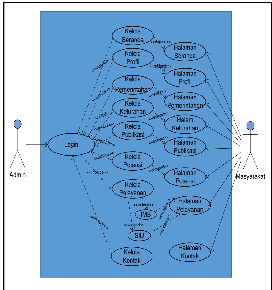
Gambar 5.3. Use Case yang diusulkan
