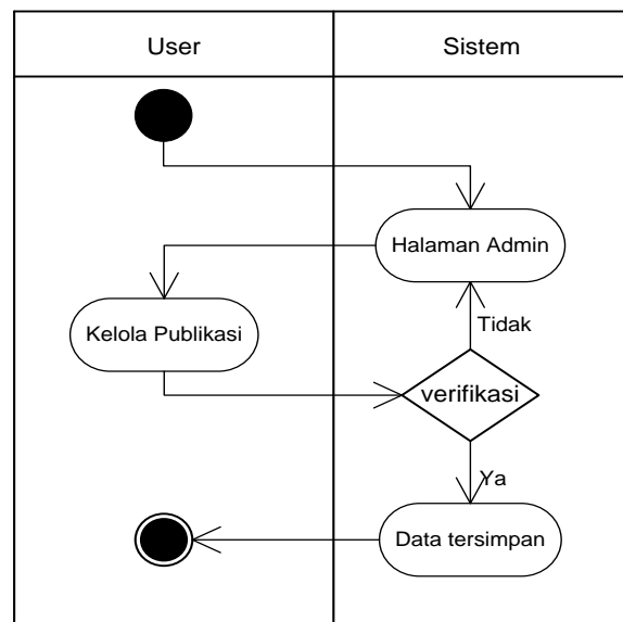
Gambar 5.9. Activity Diagram Kelola Publikasi
