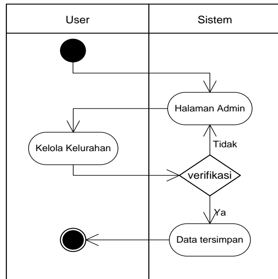
Gambar 5.8. Activity Diagram Kelola Kelurahan
